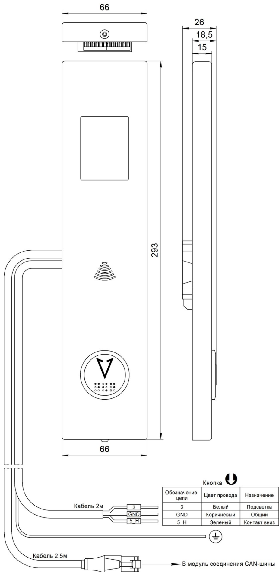
Рис.1 Внешний вид, габаритные и установочные размеры Вызывного поста ВП-1102Е-1086-11 (жгут RJ45)
